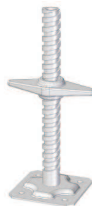
Socle à vis/ Regelbare voet
